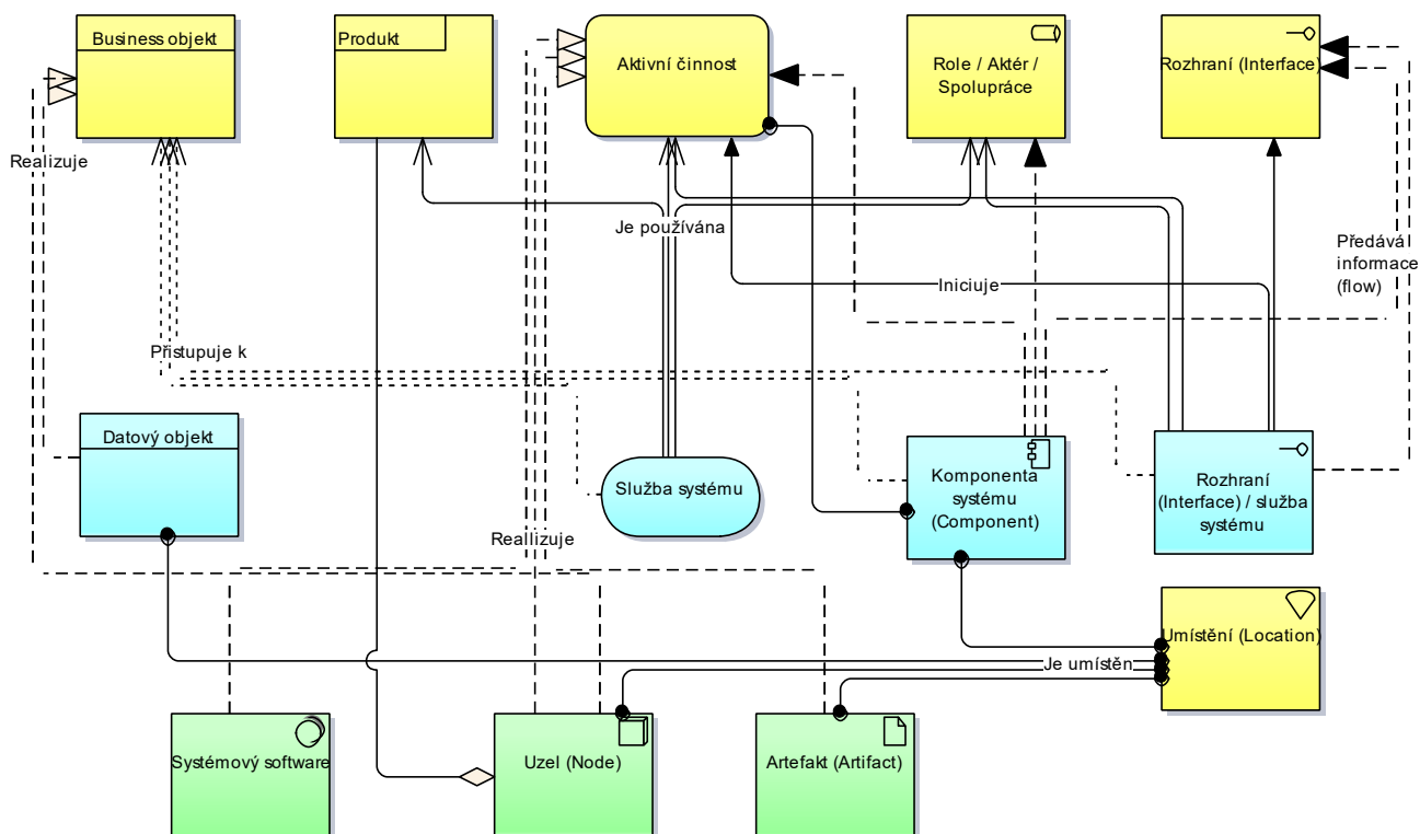
Obrázek 15 Vertikální vazby business vrstvy na nižší vrstvy
