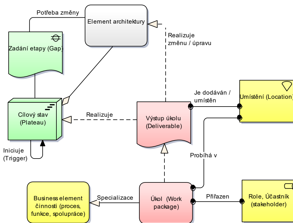
Obrázek 20 Metamodel rozšíření Implementace s vazbami na Enterprise architekturu
