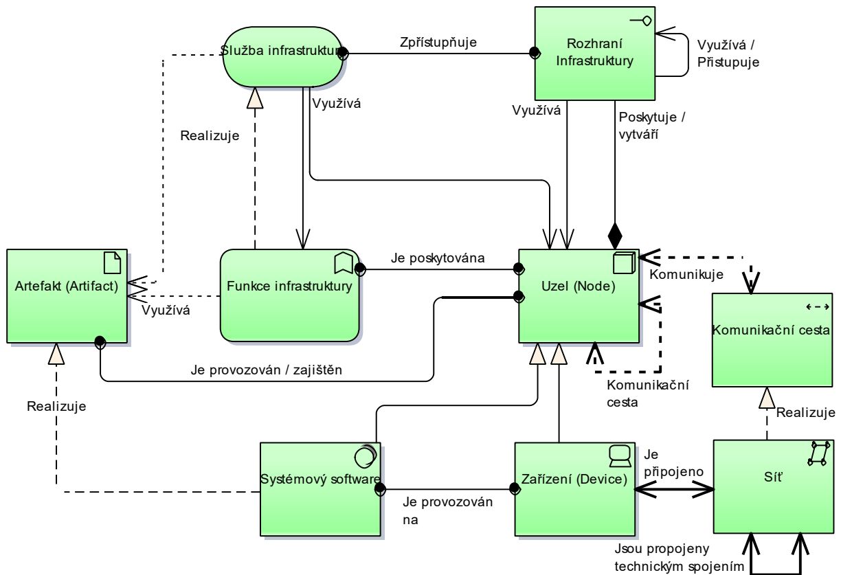
Obrázek 9 Metamodel technologické vrstvy - informační model
